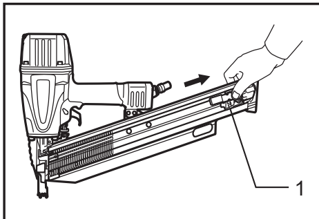
► 1. Poussoir
