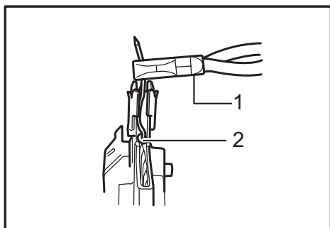
► 1. Pliers 2. Slot
