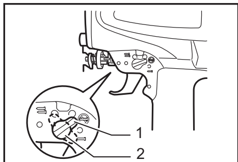
► 1. Verrou de la gâchette 2. Levier de changement
